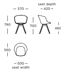
Mono V3 Wooden base
