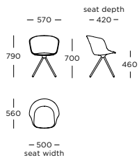
Mono V1 Spider base
